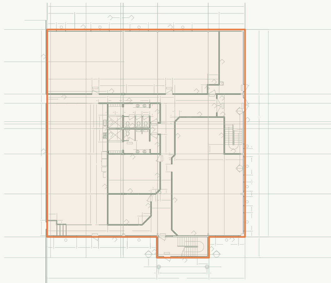
1층 평면과 검토용 외곽
